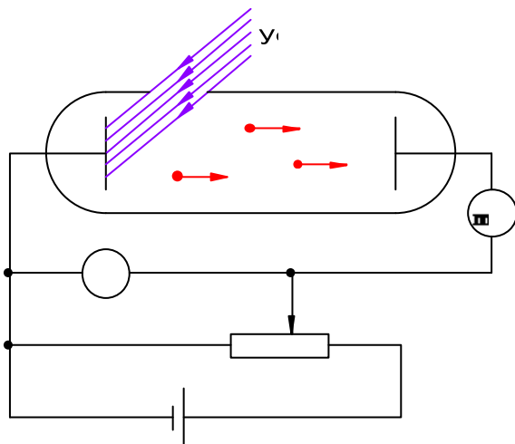
Рис. 1. Фотоэлемент Столетова
